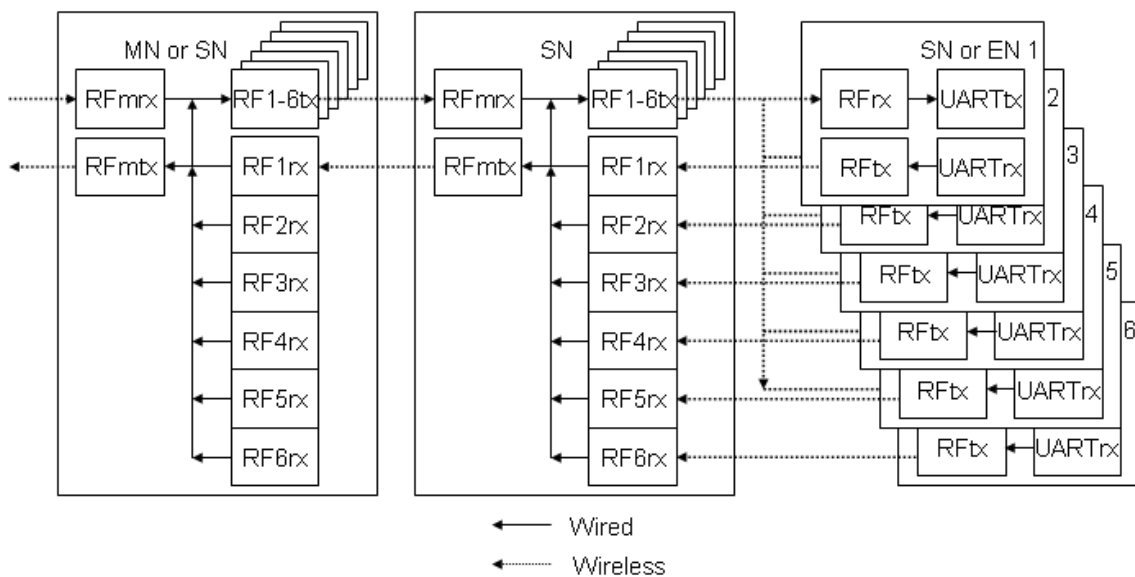
그림 2-12 MN HUB-SN HUB-EN Data Flow
