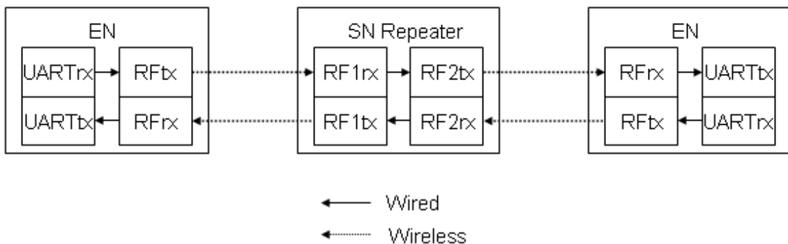
그림 2-6 EN-SN Repeater-EN Data 흐름
