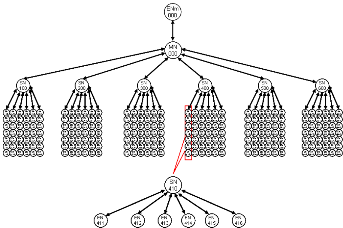
그림 3-6 260 Node Master-Slave
