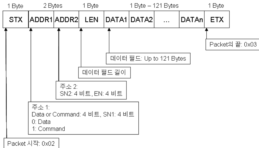
그림 2-3 Address Mode의 Packet 구조
