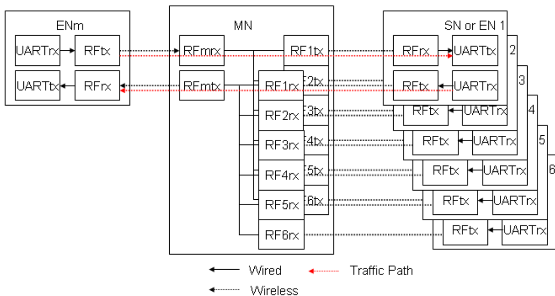
그림 2-14 MN Unicast-SN Unicast-EN Data Flow
