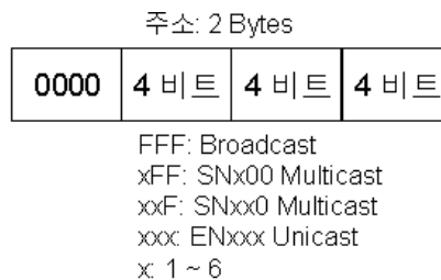
그림 2-4 Packet의 Address 구조
