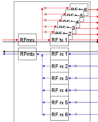
그림 2-13 MN Unicast 및 SN Unicast의 Data Routing
