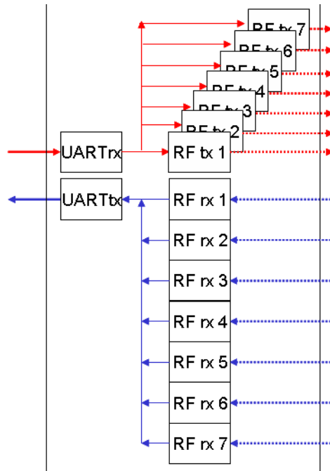
그림 2-15 UART Mode ON에서의 MN의 Data Routing
