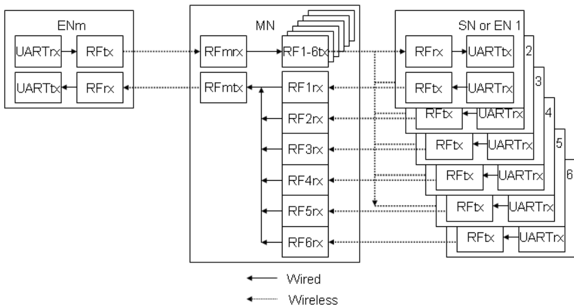
그림 2-8 EN-MN-SN 또는 EN Data Flow
