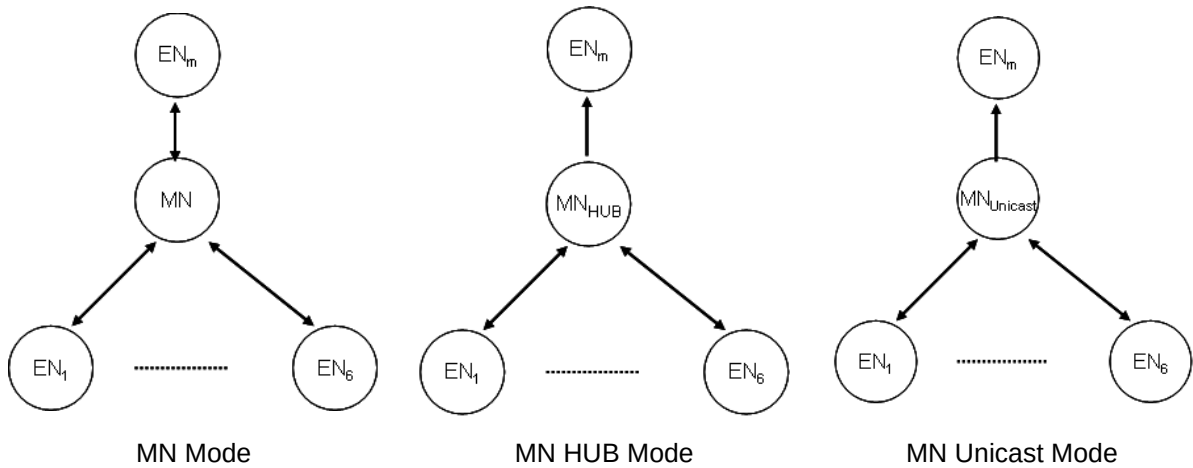
그림 3-4 7 Node Master-Slave
