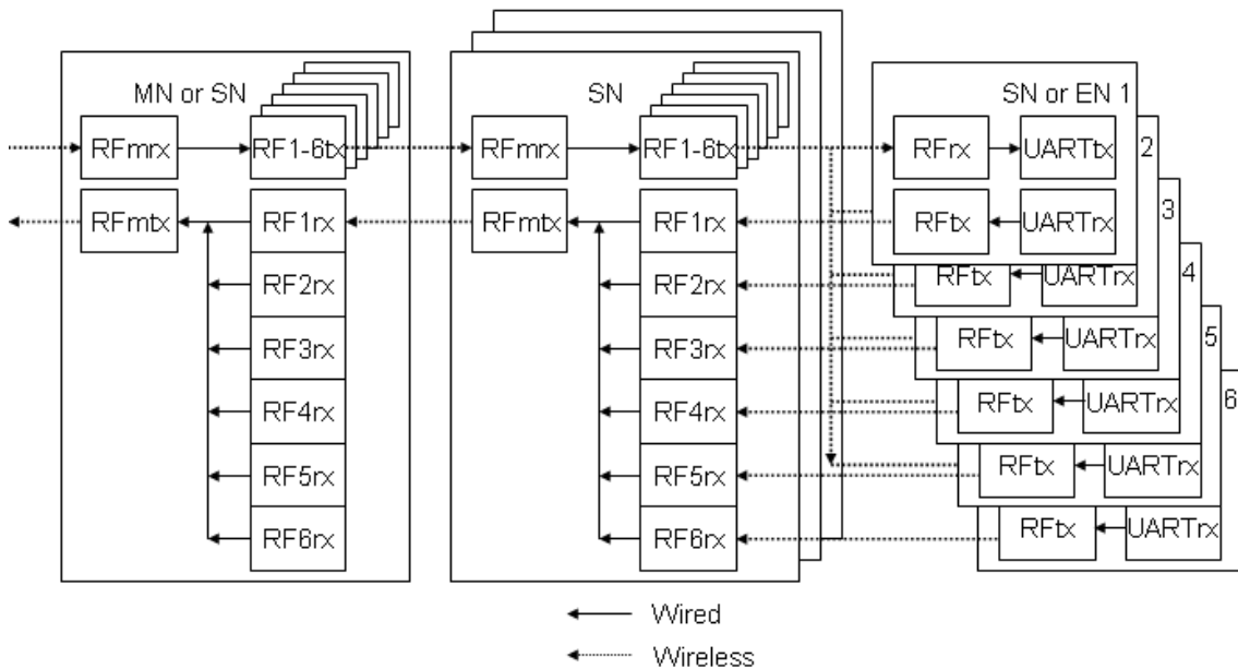
그림 2-10 MN 또는 SN-SN-SN 또는 EN Data Flow
