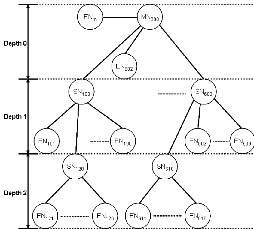
그림 3-5 Tree 구조
