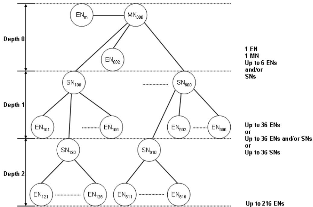
그림 2-1 Tree 구조
