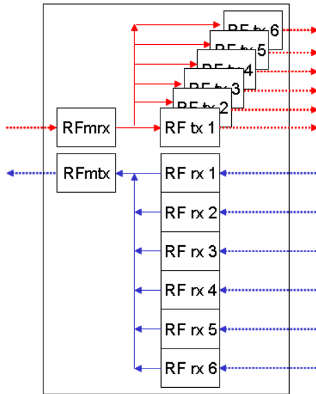
그림 2-9 SN의 Data Routing
