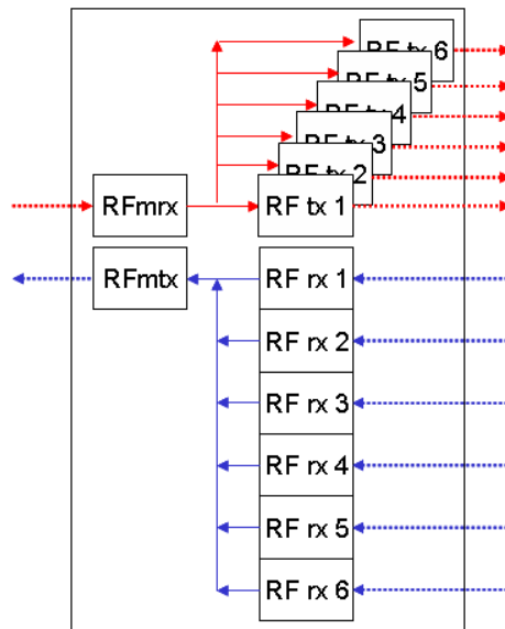
그림 2-7 MN의 Data Routing
