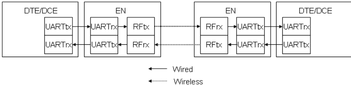
그림 2-5 EN-EN Data 흐름
