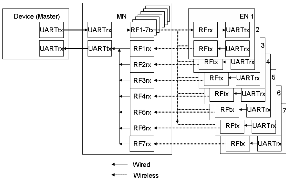
그림 2-16 UART Mode ON에서의 MN-EN Data Flow
