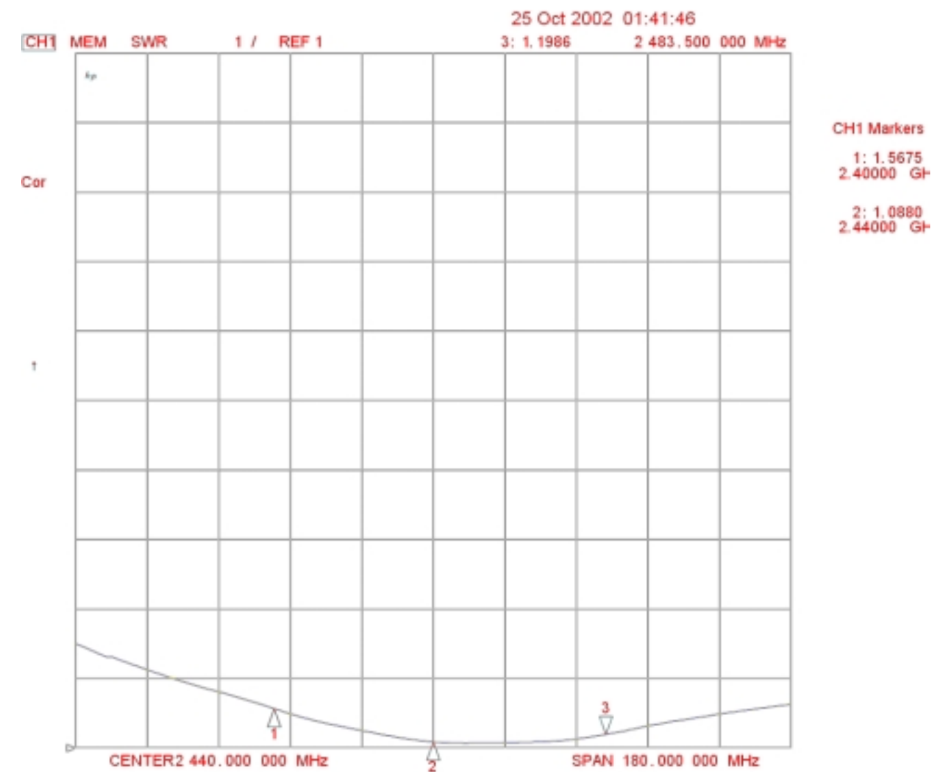
Fig 1. VSWR
